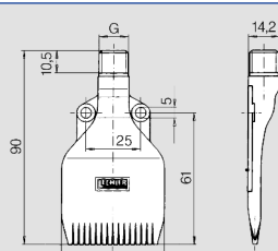
Weight: 23 g · T max POM: 50 °C Weight: 15 g · T max PP: 60 °C
