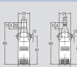
Weight: 16 g · T max : 50 °C
