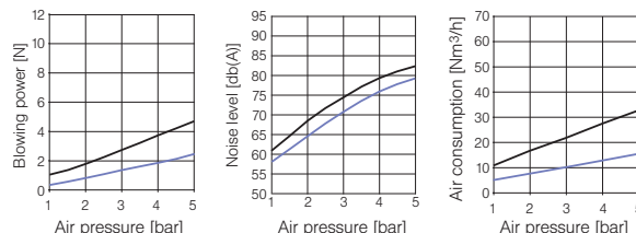
— Type 600. 130 — Type 600. 484
